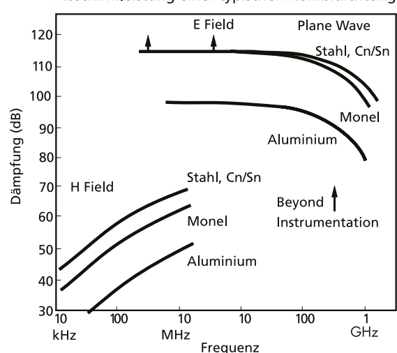
Abschirmleistung einer typischen Kombidichtung
